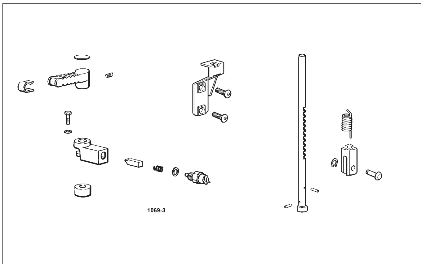
Fig. 8 - Handbrake control.
