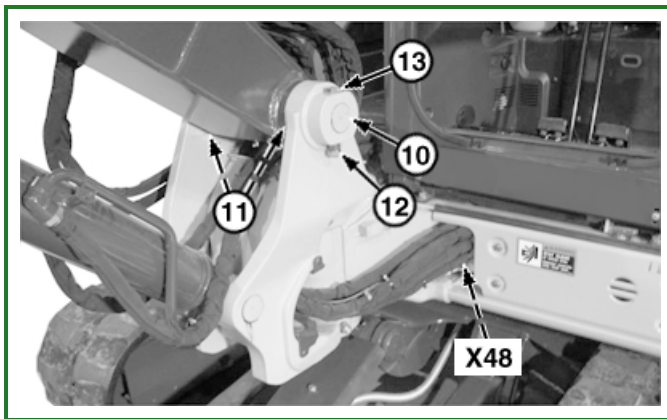
TX1134540A-UN: Boom Pin
